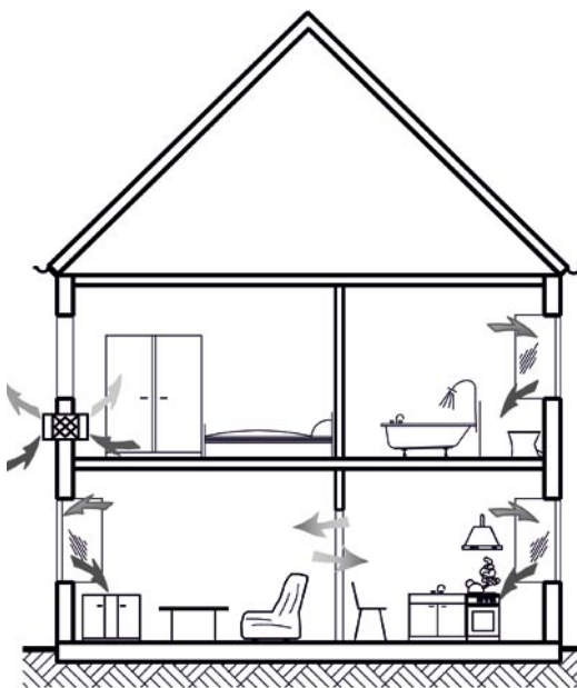
Bild 12: Ventilatorgestützte Lüftung: Dezentrales Lüftungsgerät (■ und ■ = Abluft; ■ und ■ = Zuluft)
