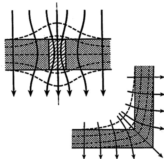
Bild 4: Schematische Darstellung zweier Wärmebrücken mit Angabe der Wärmeströme (Adiabaten; durchgezogene Linien) und Isothermen (gestrichelte Linien). Wärmebrücken zeichnen sich physikalisch durch verstärkten Wärmefluss mit Verdichtung der Adiabaten und Wölbung der Isothermen aus (nach Gertis et al. 2001)
