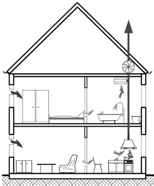
Bild 10: Ventilatorgestützte Lüftung: ALD und Abluftanlage (■ = Abluft; ■ = Zuluft)
