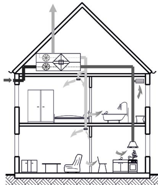
Bild 11: Ventilatorgestützte Lüftung: Zu- und Abluftanlagen (■ und ■ = Abluft; ■ und ■ = Zuluft)
