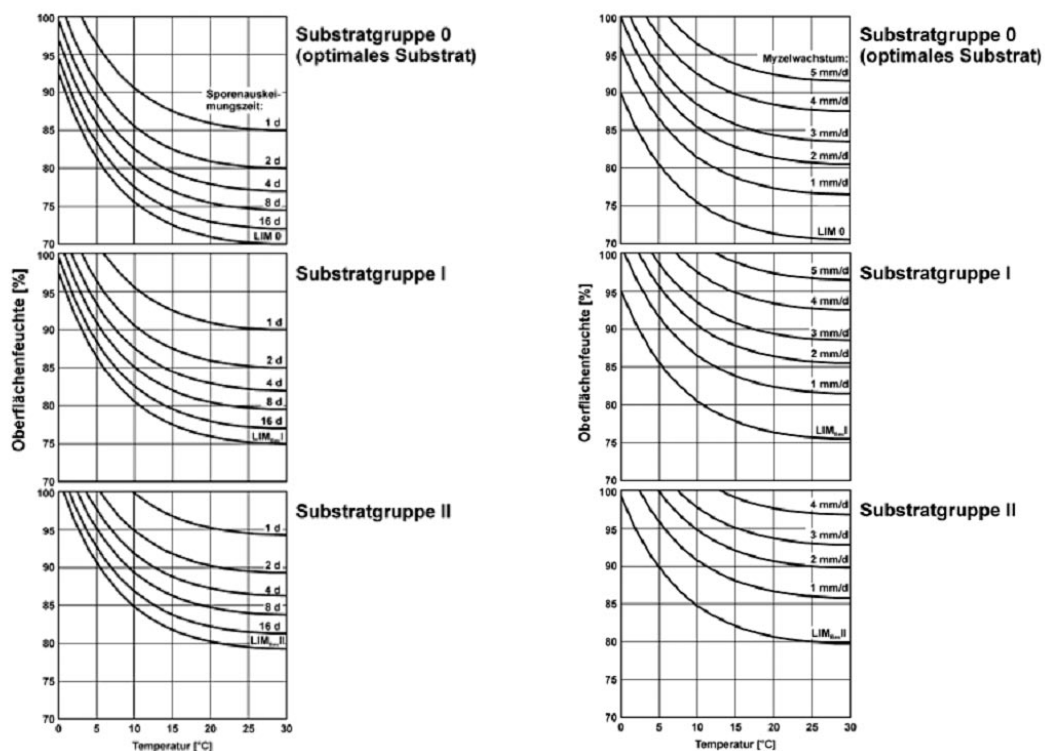
Bild A: Verallgemeinertes Isoplethensystem für die Sporenauskeimung , das für alle in Bauteilen auftretenden Pilze gilt (nach Sedlbauer 2001); Bild oben gilt für optimales Substrat, Mitte für Substratgruppe I und Bild unten für Substratgruppe II. Die angegebenen Werte charakterisieren die Zeitdauer, nach welcher eine Keimung abgeschlossen ist. LIM = Lowest Isopleth for Mould = unterste Grenze der Sporenauskeimung
